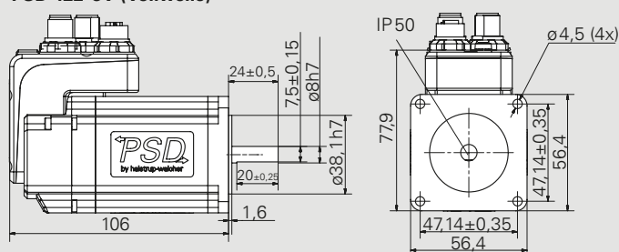
PSD 432-8 / 14H (Hohlwelle, 2 und 4 Nm)
