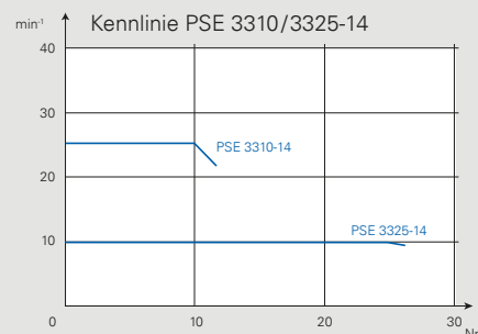
Kennlinie PSE 3310/3325-14
