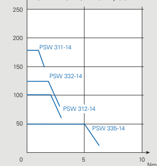
Kennlinie PSW 31x/33x-14
